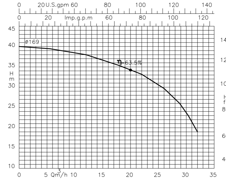
ETA BLOCK 32-160
