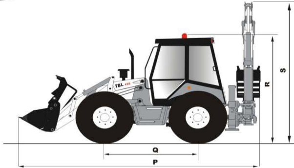
ابعاد کلی
